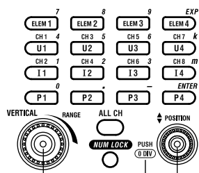
RANGE knob
