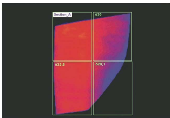
Darstellung von Heizzonen im Wärmebild einer Glasscheibe
